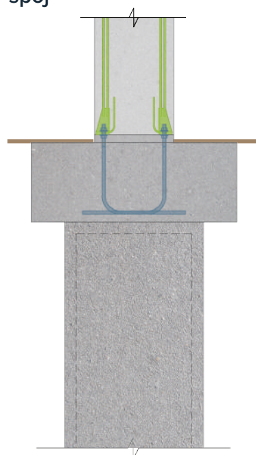
Šroubový spoj na základové patce/pilotové hlavici
