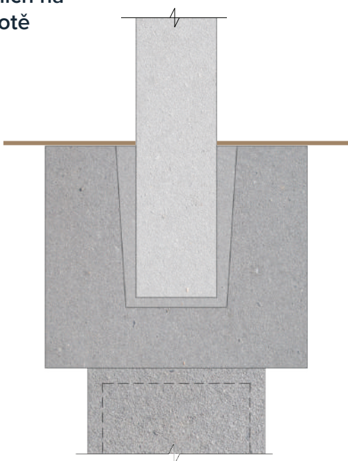
Kalich na základové patce/pilotové hlavici
